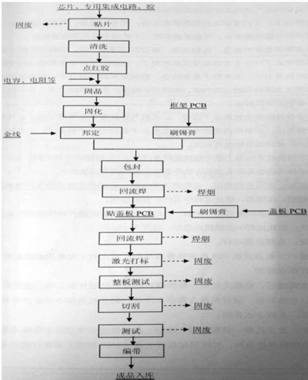
图5.1原工艺流程图
